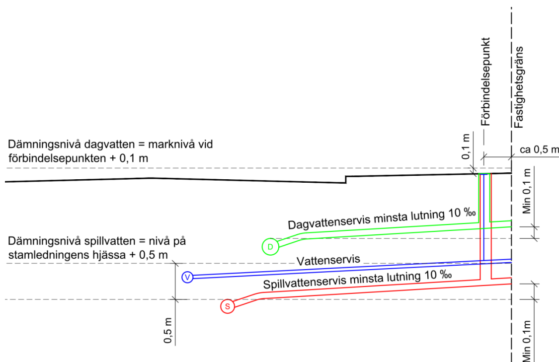
Figur 3.6 Sektion A-A vattengångsnivåer på servisledningar i förbindelsepunkt och dämningnivåer
